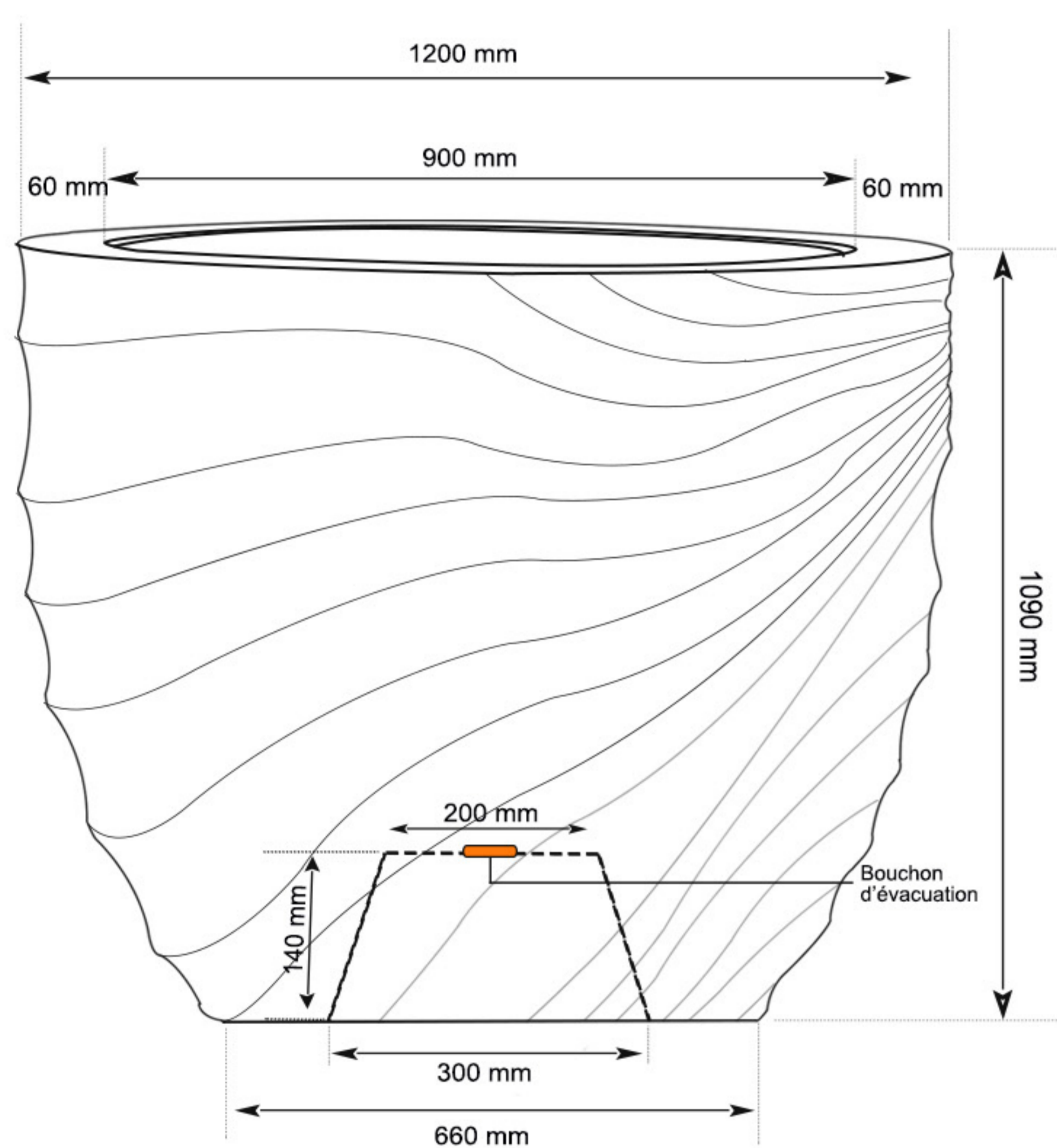
DUNE-1200 Poids : 33 kg Volume : 1000 L
